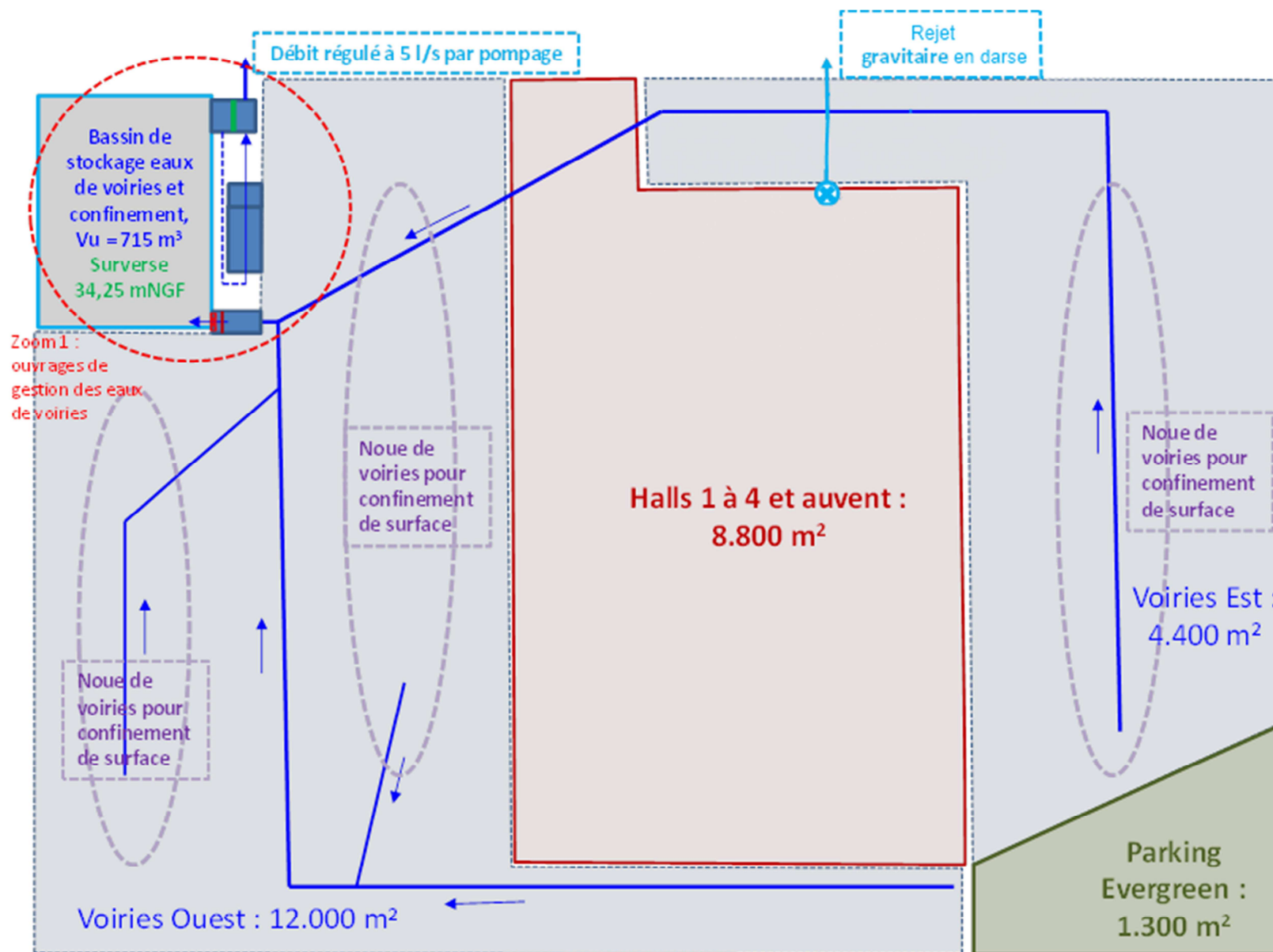
Figure : Extrait étude de dimensionnement des ouvrages de gestion des EP du site – organisation générale de la gestion des eaux pluviales
